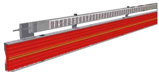
Exemple d'application de système Pro-Ductor avec positionnement au moyen d'une bande à code barres.
