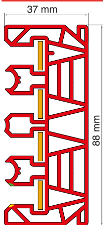
Profil PR4 avec conducteurs
