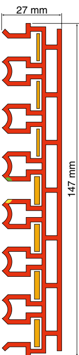
Profil PR7 avec conducteurs
