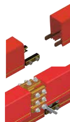
Montage de la pincette de raccordement Cu-S
