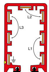
Gaine RC7, standard à 7-pôles bandes parallèles
